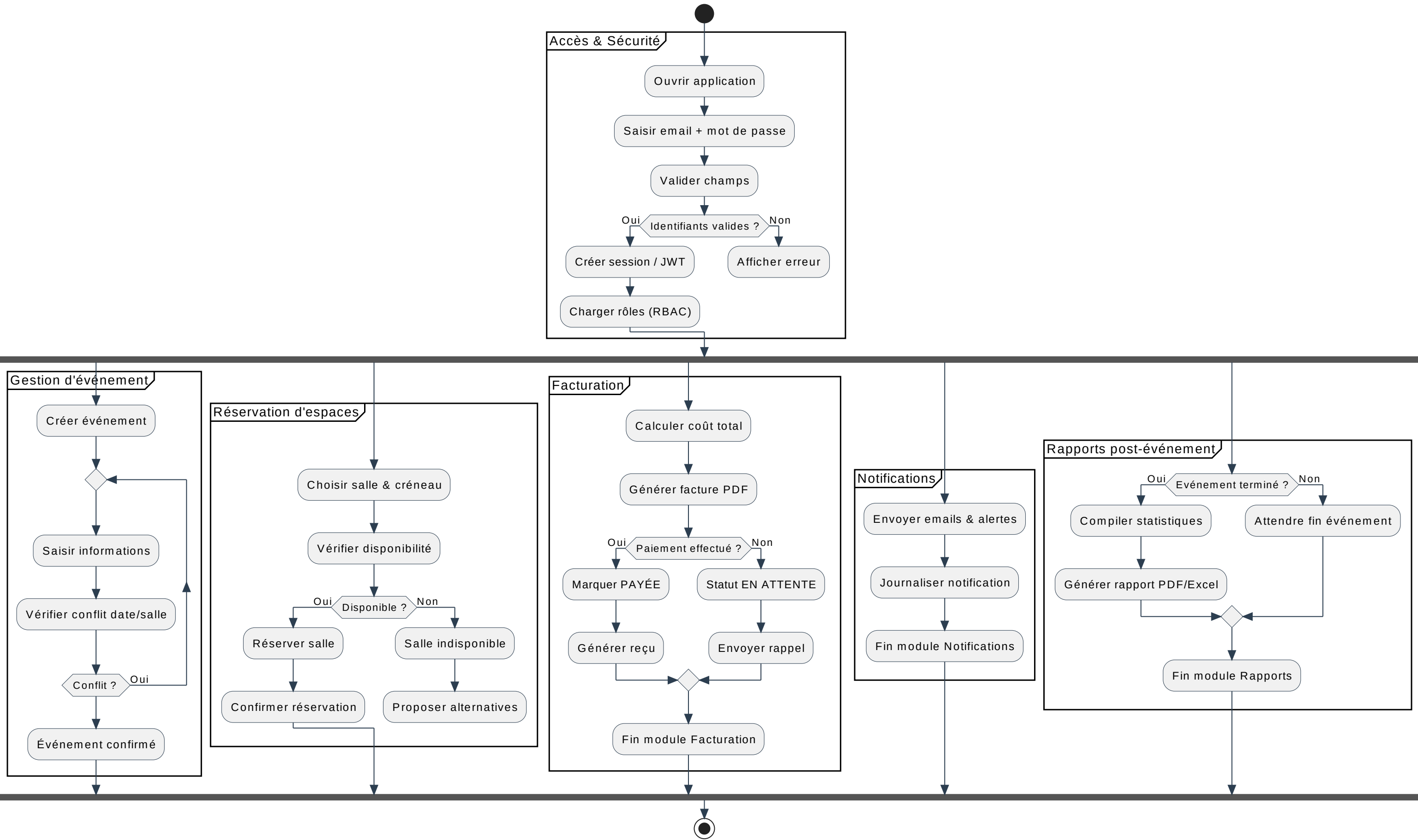
Diagramme d'activité - Plateforme de gestion d'événements
